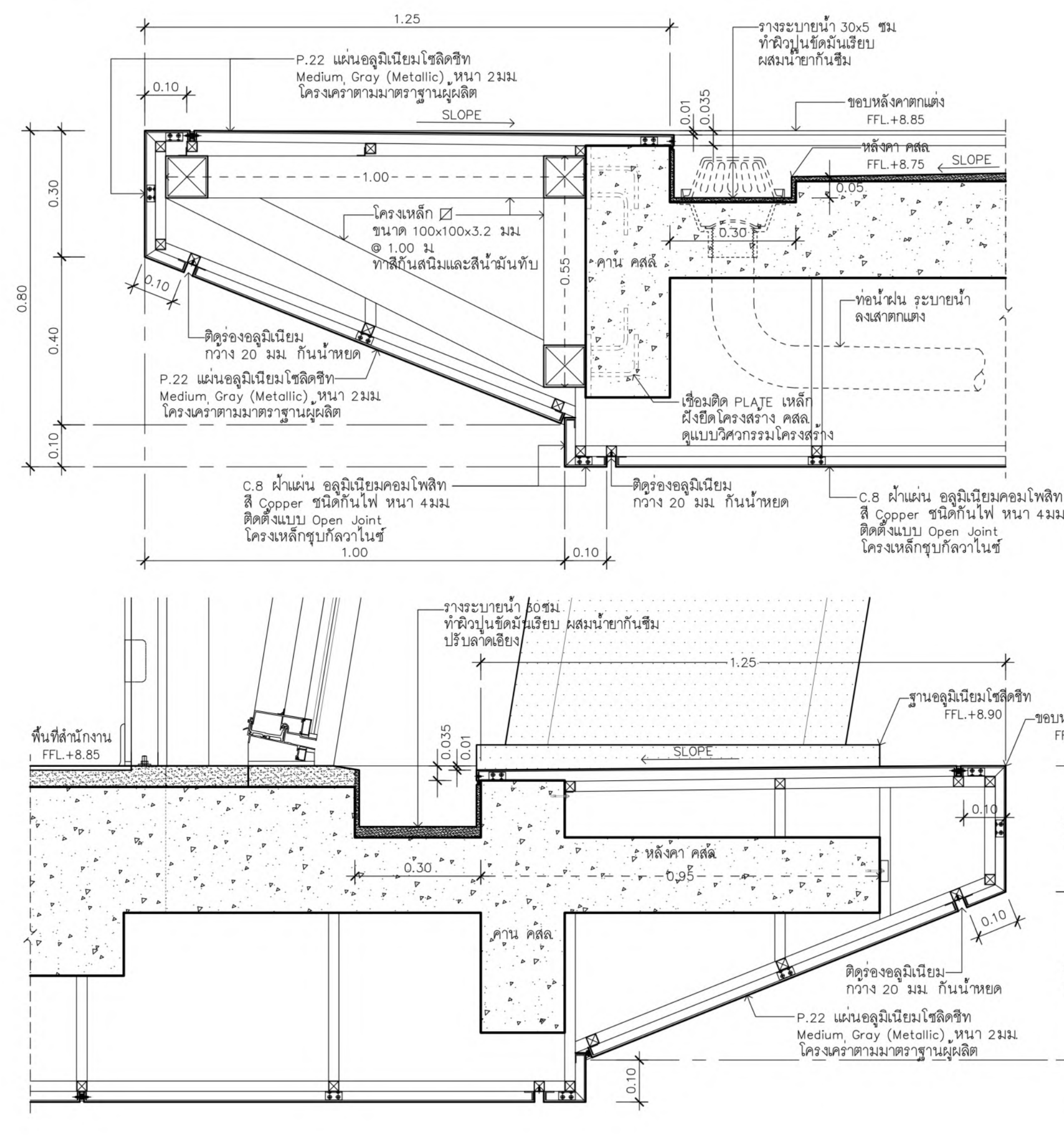
แบบขยายปลายหลังคา 2
