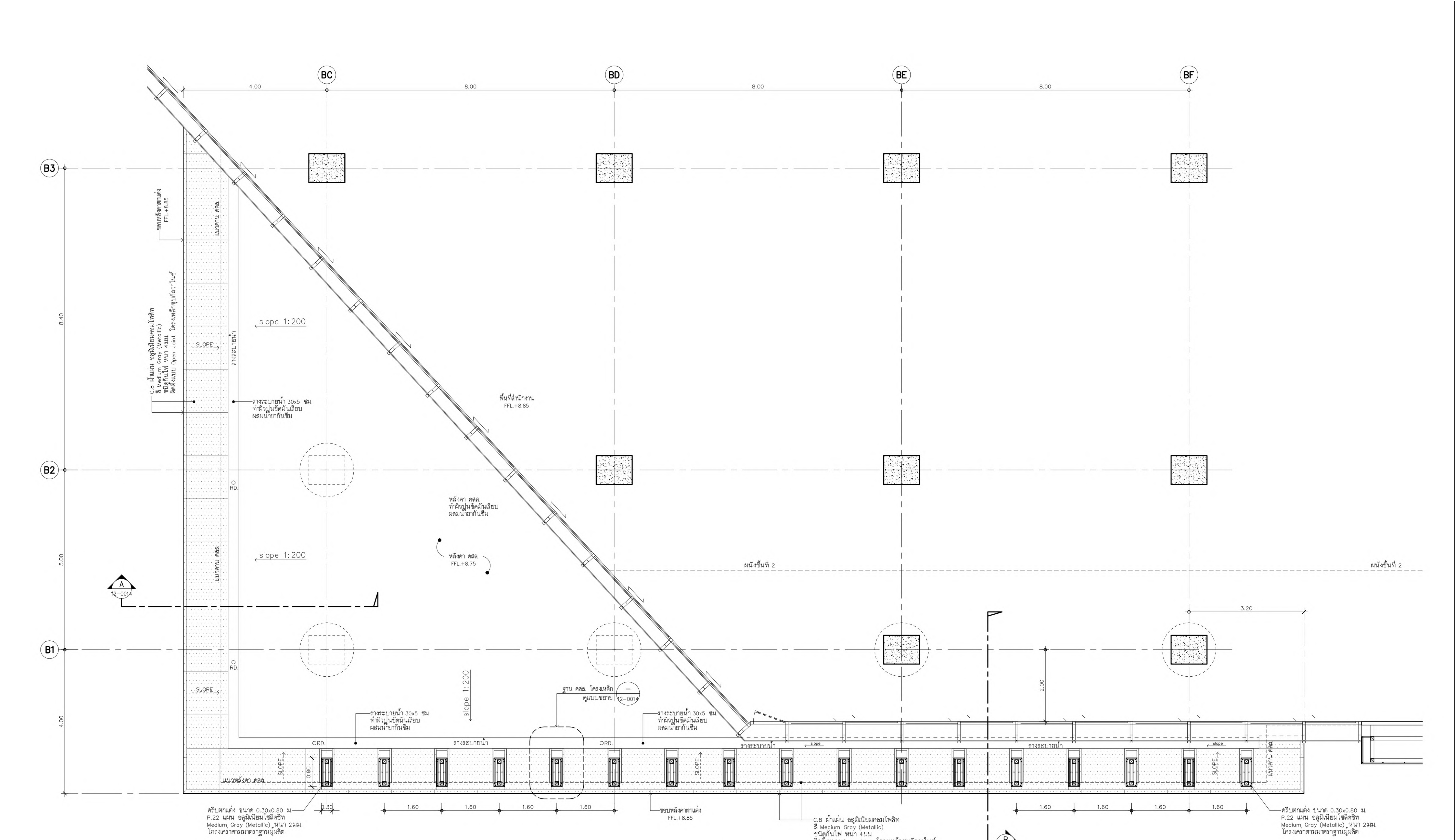
แปลนขยายหลังคา CANOPY 3 มาตราส่วน 1:50 ระดับพื้นที่ 3
