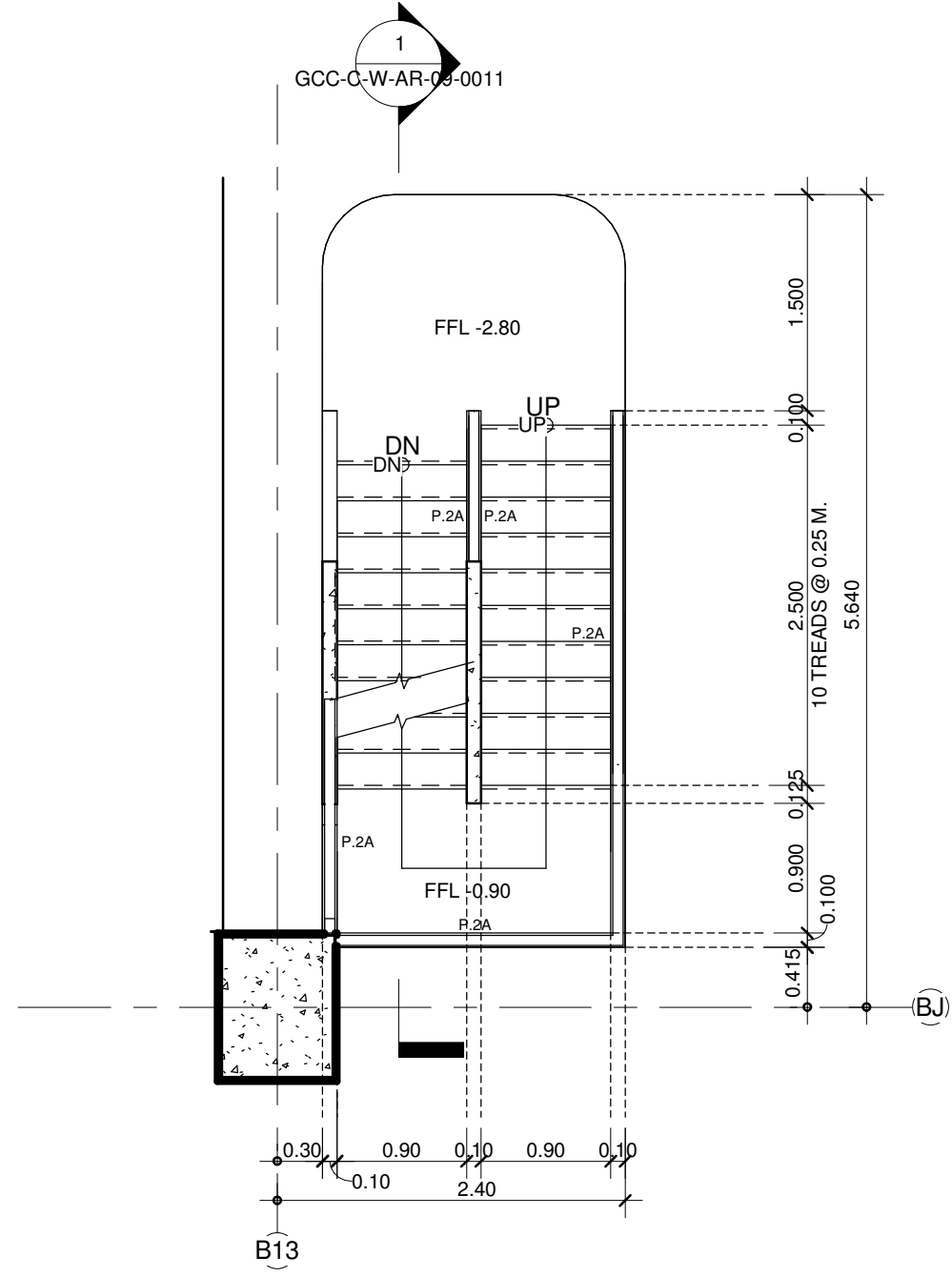
แบบขยายบันได WST.03b ชั้น B1 1 : 50
