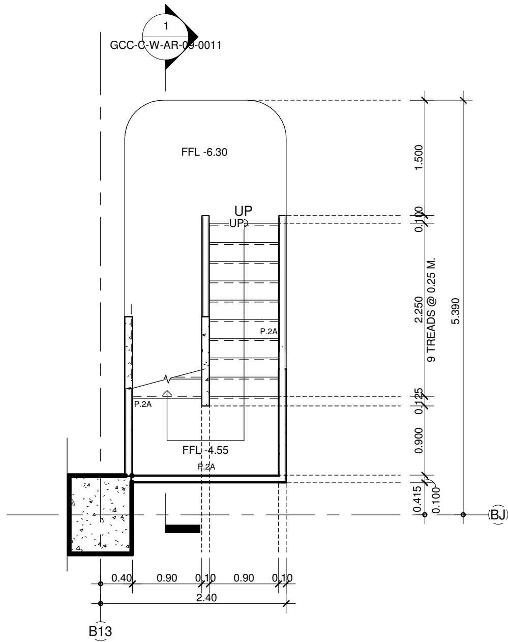
แบบขยายบันได WST.03b ชั้น B2 1 : 50
