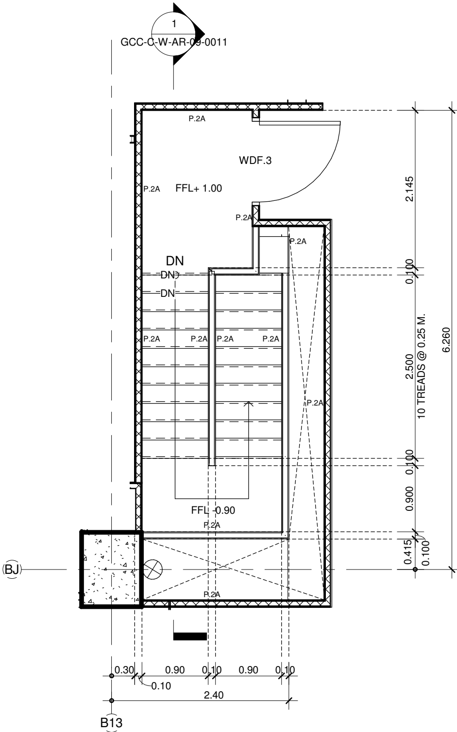
แบบขยายบันได WST.03b ชั้น 1 1 : 50
