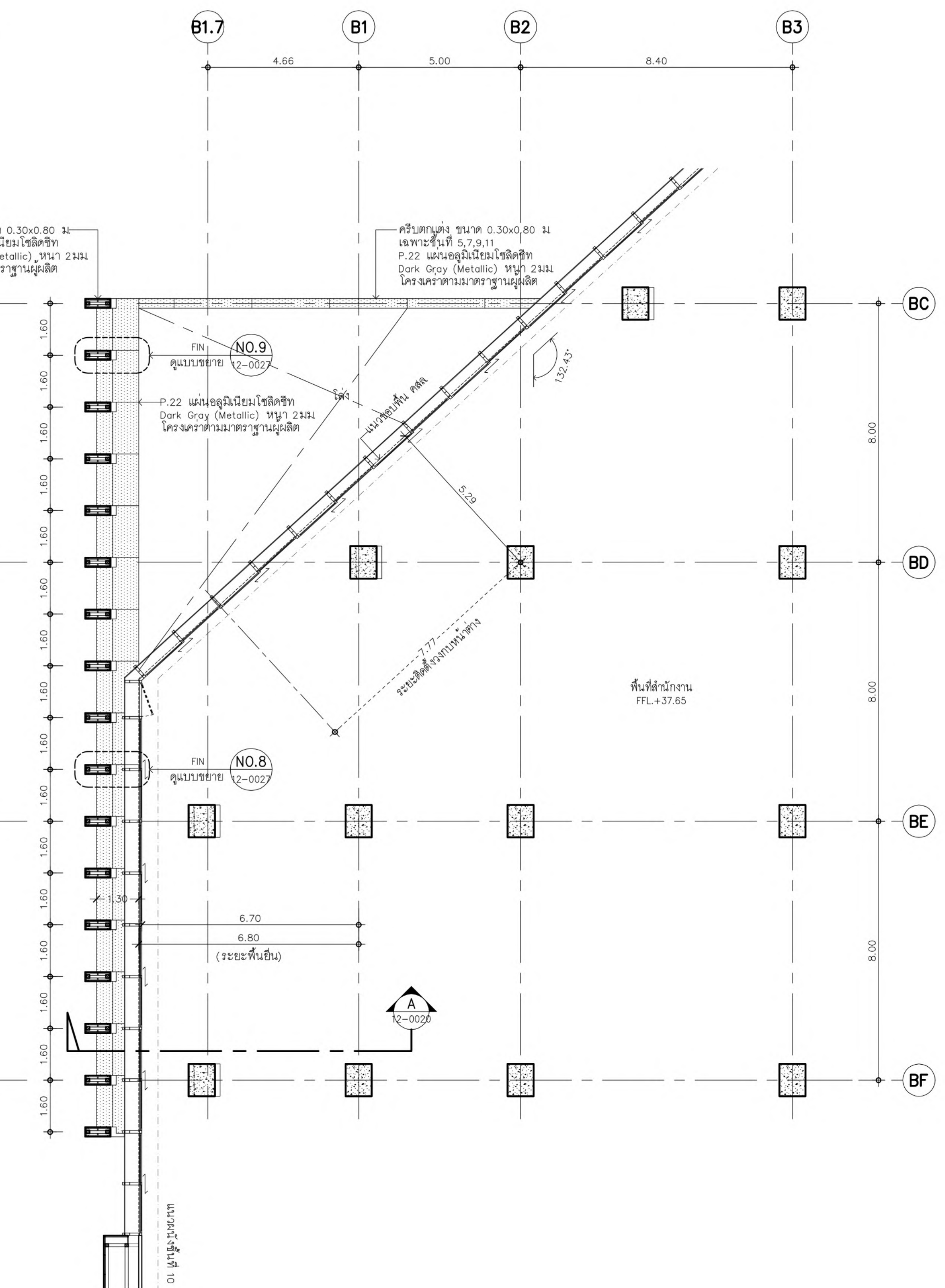
แปลนขยายครีบทกแต่ง 1
